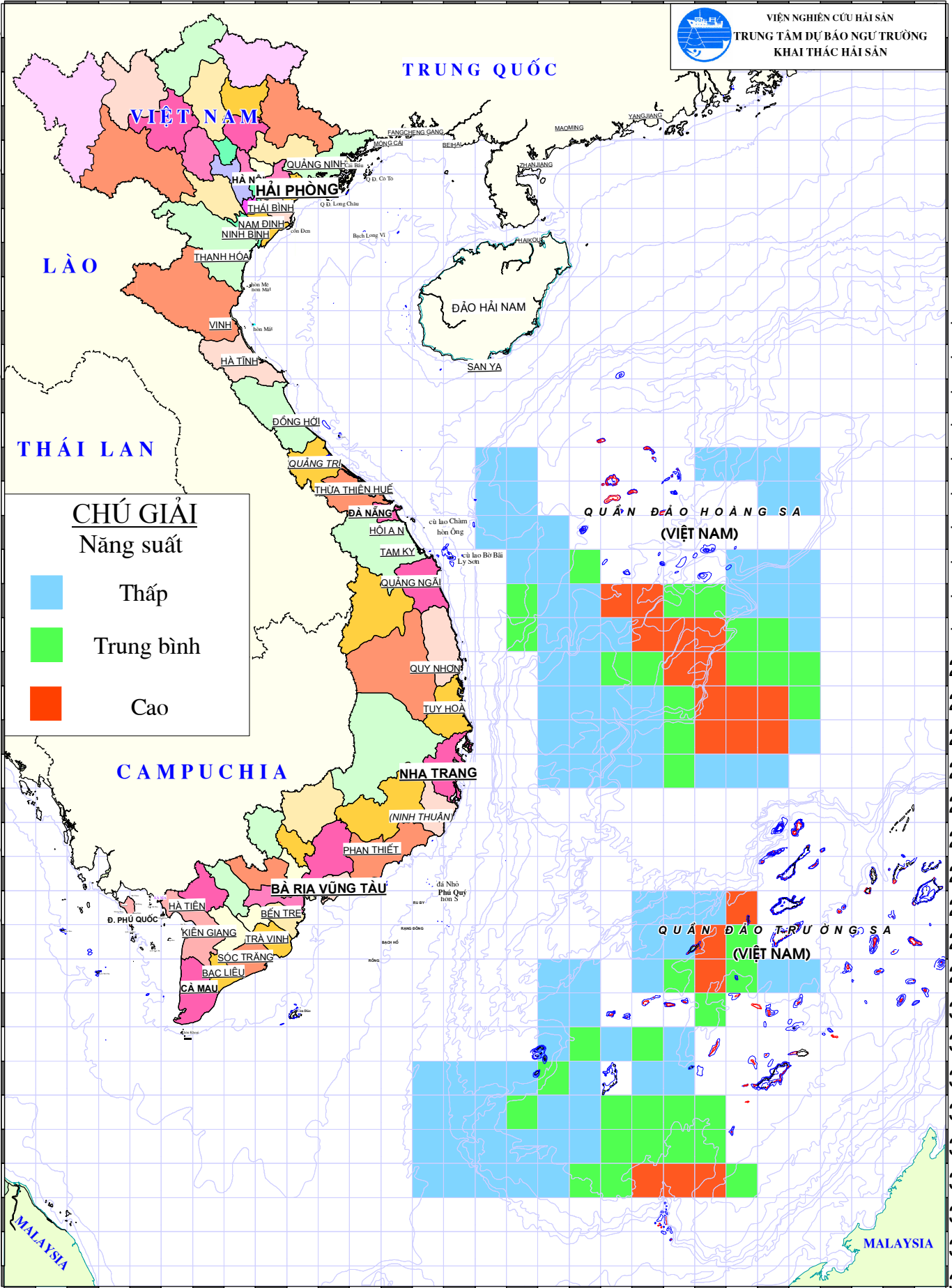
BẢN DỰ BÁO NGƯ TRƯỜNG KHAI THÁC CÁ NGỪ ĐẠI DƯƠNG TỪ NGÀY 24 ĐẾN 30 THÁNG 09 NĂM 2017
