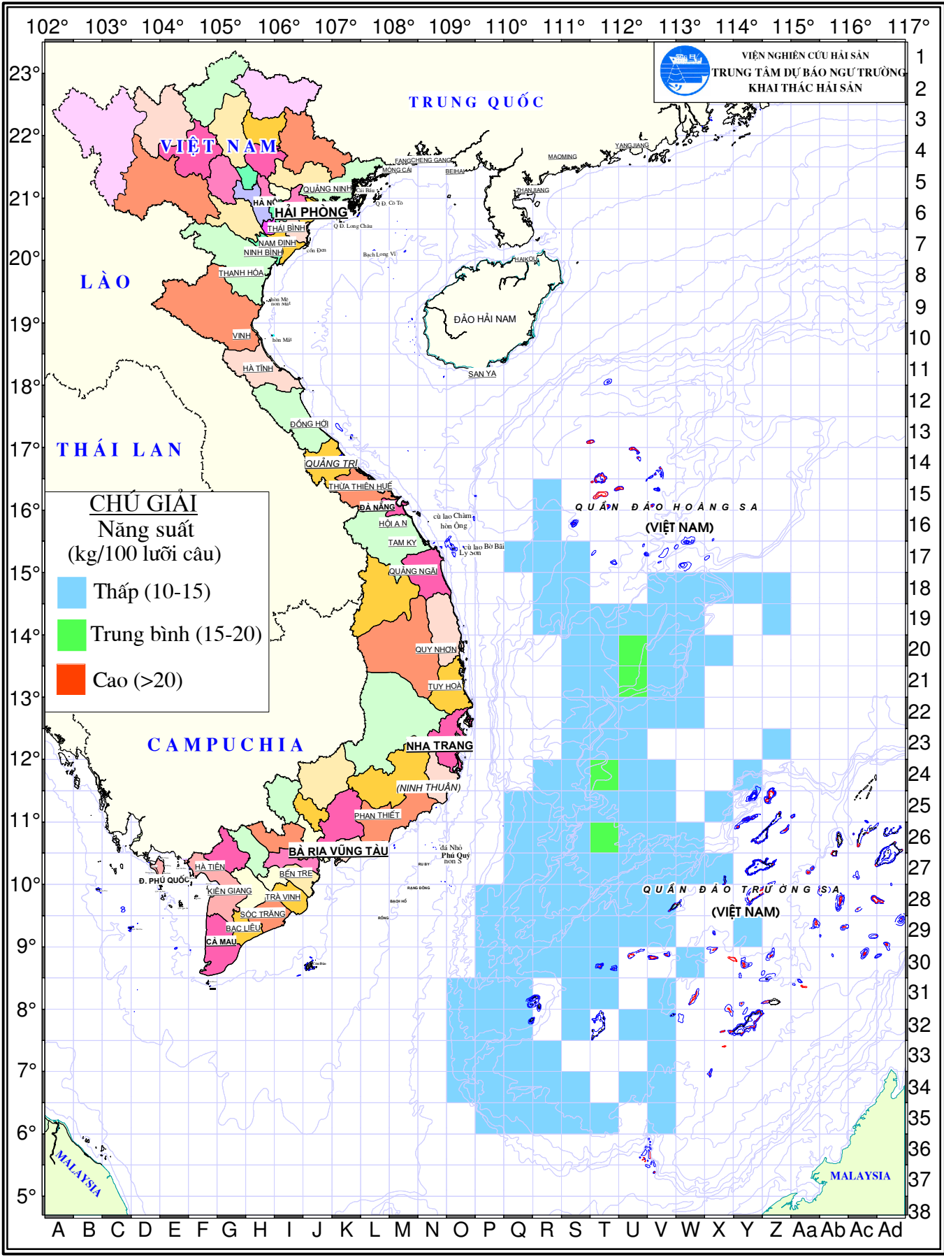
BẢN DỰ BÁO NGƯ TRƯỜNG KHAI THÁC NGHỀ CÀU CÁ NGỪ ĐẠI DƯƠNG TỪ NGÀY 01 ĐẾN 10 THÁNG 07 NĂM 2016
