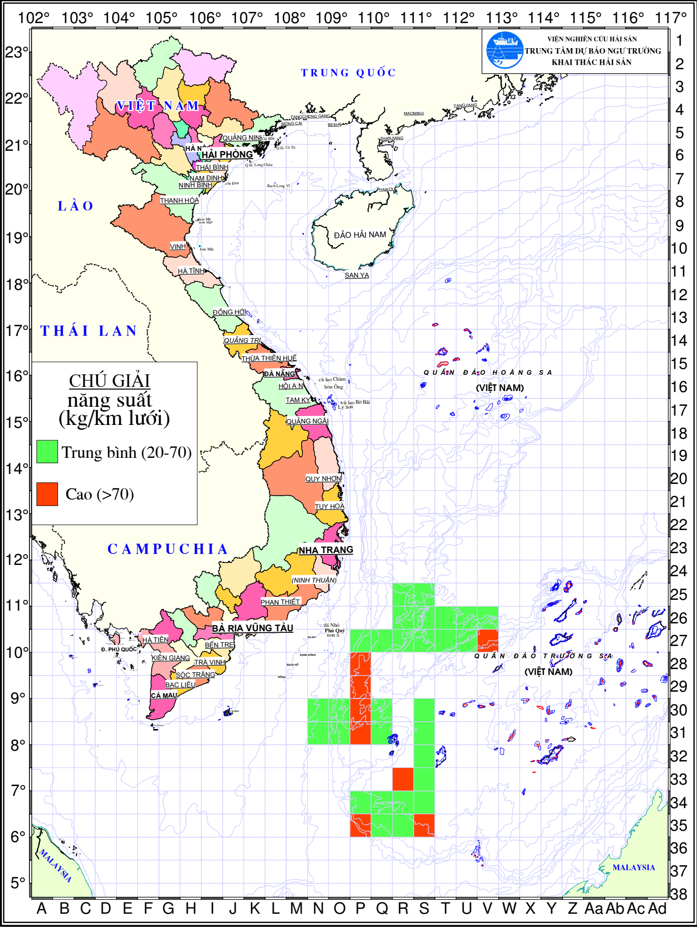
BẢN DỰ BÁO THỬ NGHIỆM NGƯ TRƯỜNG KHAI THÁC CÁ NGỪ VẦN THÁNG 12 NĂM 2016
